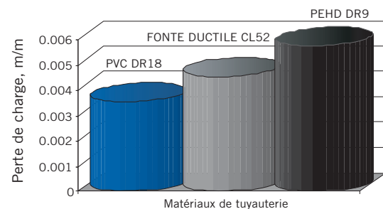
Perte de charge - Tuyau de 200 mm à 25 L/s
